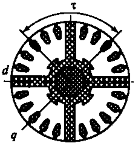
Сегментный ротор
